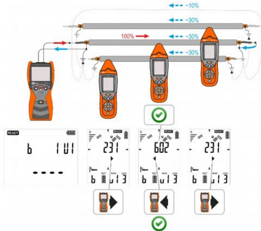
Идентификация кабельной линии с помощью приёмника LKO-720
