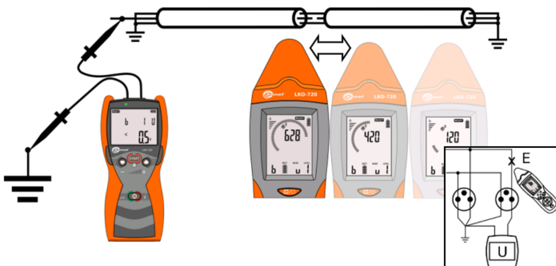
Поиск места разрыва
