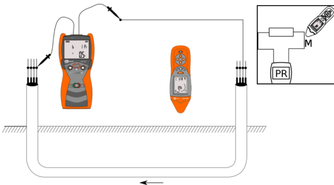
Поиск кабельной линии с замкнутыми жилами в режиме «мощность»
