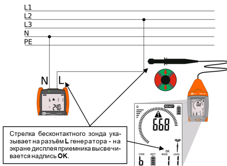
Идентификация разъёма L генератора
