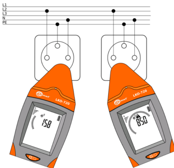
Обнаружение электрического поля
