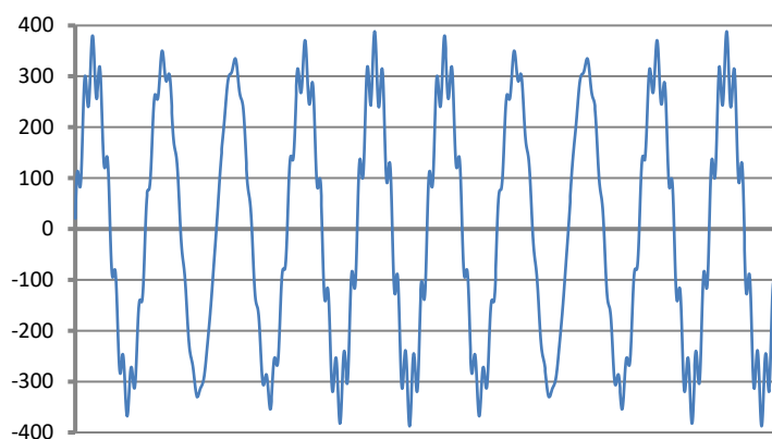
Рис.47. Эффект взаимодействия 9-й гармоники (450 Гц, 10% U_{ном} ) и интергармоники 460 Гц (10% U_{ном} ). Видимые изменения формы напряжения с частотой 10 Гц, которые могут создать эффект мерцания света ( U_{ном} = 230 В RMS, 50 Гц).
