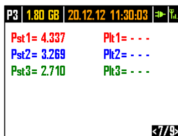
Рис.11. Экран 7/10 с показателями мерцания света.
