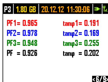
Рис.10. Экран 6/10 с коэффициентами мощности и tgφ.
