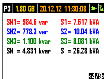
Рис.8. Экран 4/10 с мощностями искажений и полной мощностью.
