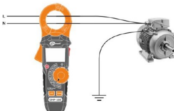
Измерение тока утечки – косвенный метод
